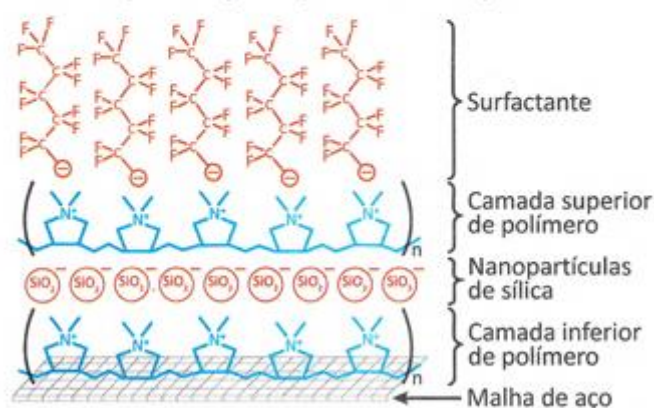
Representação esquemática do dispositivo
